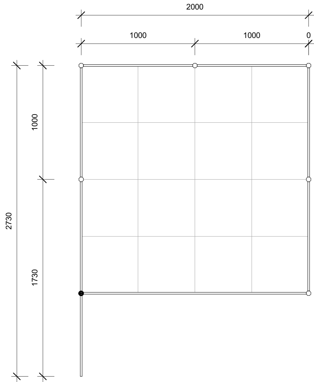
① PLAN LAYOUT 1 : 20
